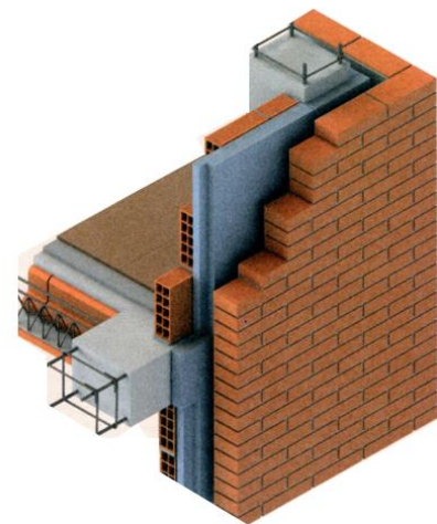
DOPPIA PARETE CON INTERCAPEDINE D'ARIA
